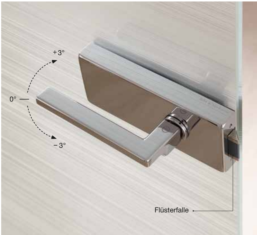
↑ Detail | Schlosskasten: Square 2.0, ähnl. Chrom Glanz
