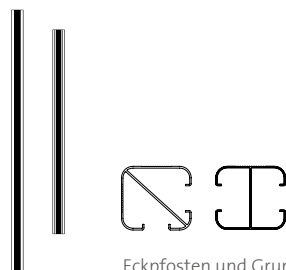
Eckpfosten und Grundpfosten
