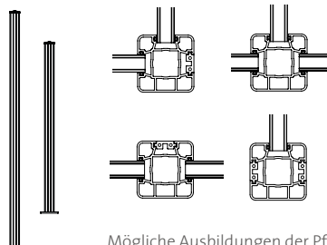
Mögliche Ausbildungen der Pfosten.
