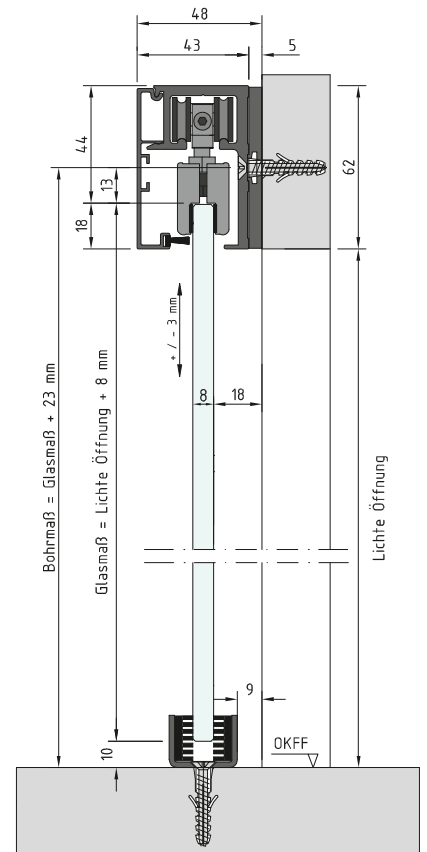
Montage mit Ganzglastür und 5 mm Hinterfütterung zur Erhöhung des Wandabstandes von 13 mm auf 18 mm, z. B. bei breiteren Sockelleisten
