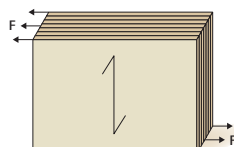
K f_{v,90,edge} hochkant, rechtwinklig♦♦
