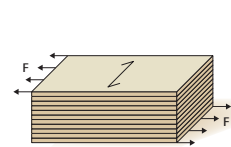
M f_{v,90,flat} und G_{90,flat} flachkant, rechtwinklig♦♦
