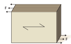
J f_{v,0,edge} und G_{0,edge} hochkant, parallel♦
