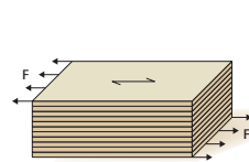
L f_{v,0,flat} und G_{0,flat} flachkant, parallel♦
