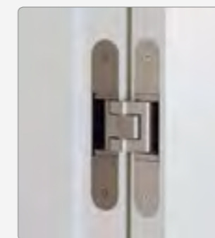
Verdecktes »Tectus« Band
