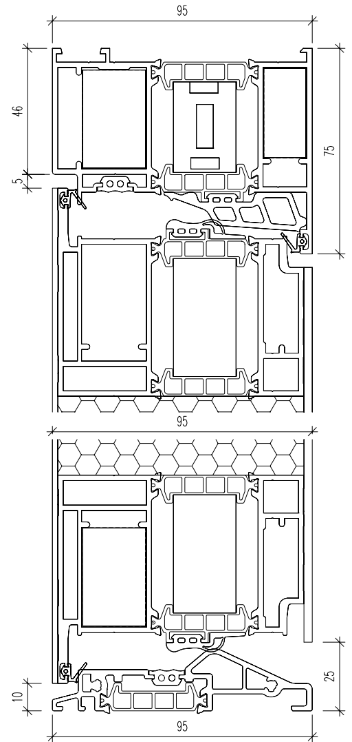
VERTIKALSCHNITT
