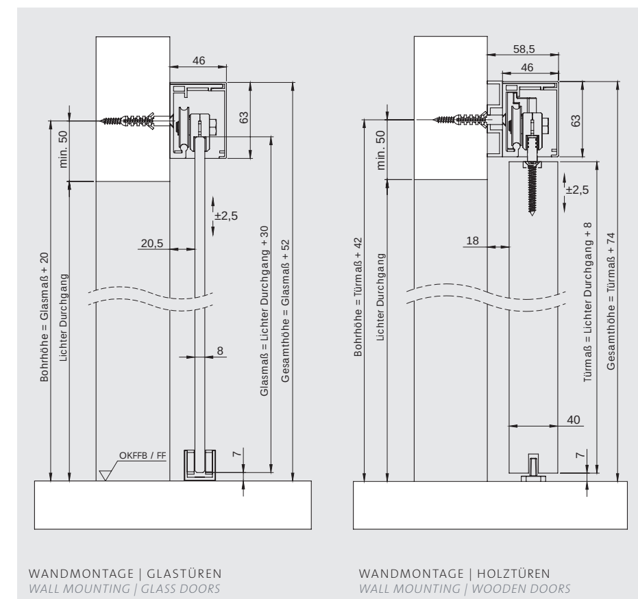
PLNEO 60 PRO WANDMONTAGE
