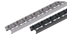
TRAGPROFIL Material: Edelstahl Normalstahl geschwärzt Länge 2000 mm
