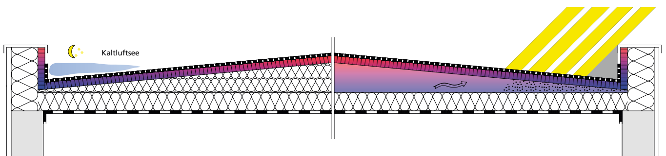
Abb. 6.6: Flachdachkonstruktionen und ihre Auswirkungen auf den Feuchteschutz: links: Entstehung von Kaltluftseen bei umlaufend hoher Attika (erhöhte Auskühlung) rechts: Strömungsverlauf in ungedämmten Hohlräumen zur Kaltseite
