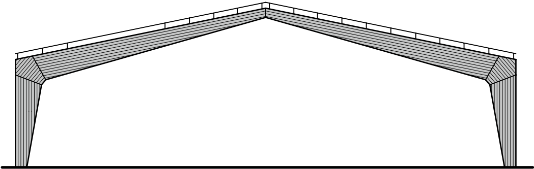
Abb. 4.2 Keilgezinkte Rahmenecken
