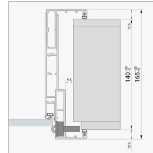
alumin impulse Umfassungszarge (rechte Tür) mit Rollenschnäpper
